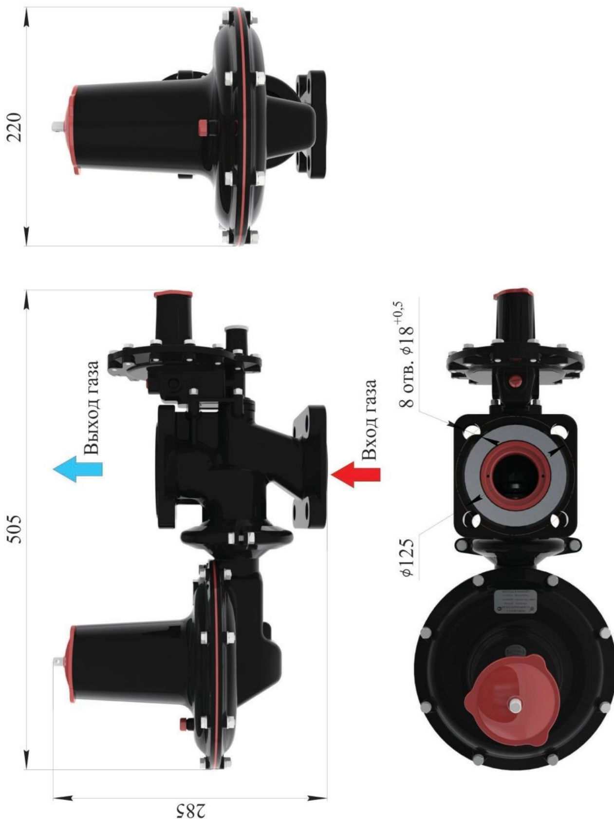
Рис. 4. Соединение фланцевое Ду 50 по ГОСТ 12817-80
