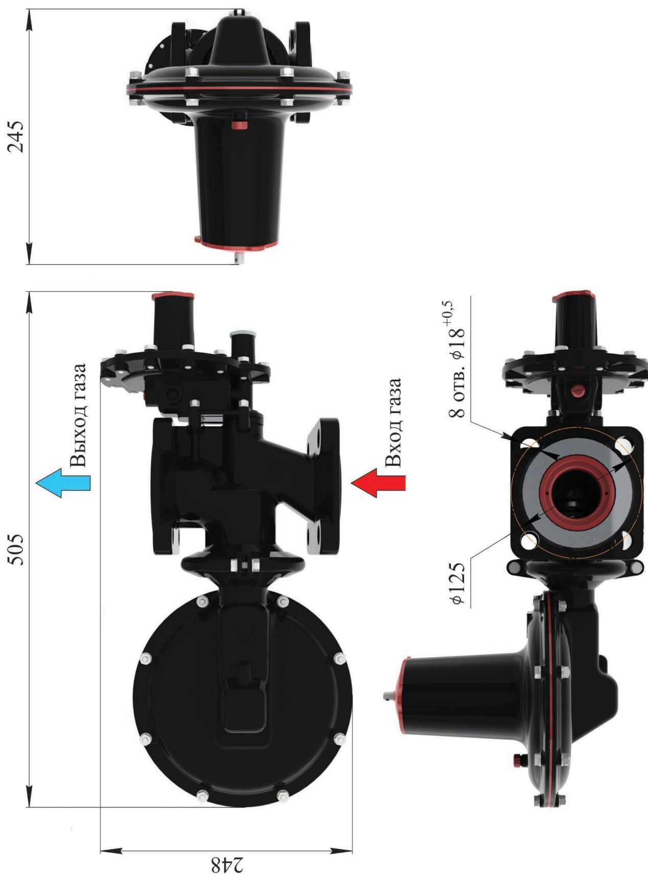
Рис. 5. Соединение фланцевое Ду 50 по ГОСТ 12817-80
