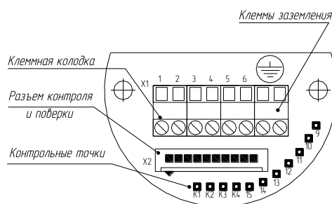
Рисунок 3 – Плата коммутации
